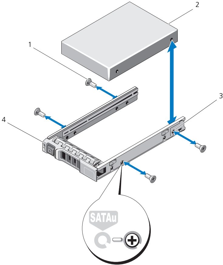
図 15-6. 2.5 インチハードディスクドライブキャリアでのハードディスクドライブの取り外しおよび取り付け
