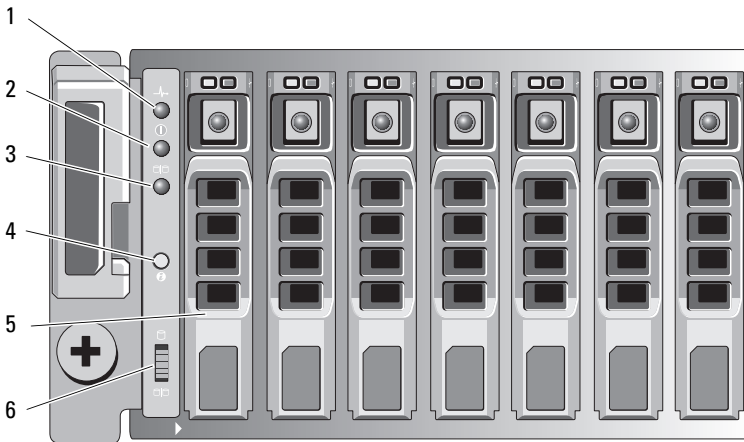
図 2-2. 前面パネルの機能およびインジケータ — Dell PowerVault MD3220
