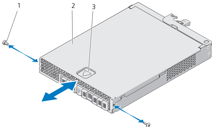
図 15-9. RAID コントローラモジュールの開閉
