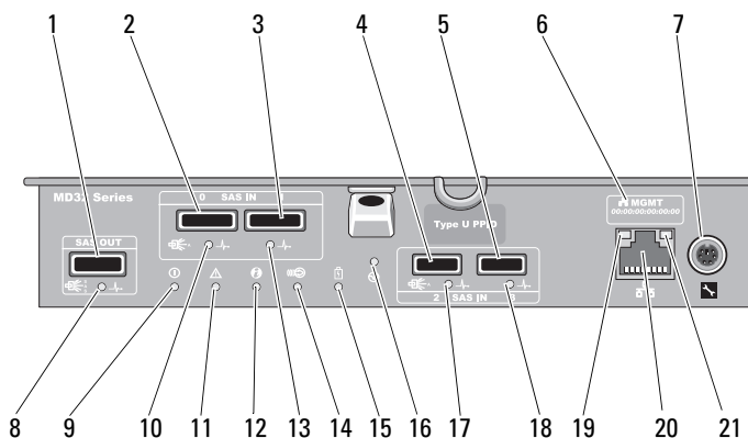
図 3-1. MD3200 シリーズ SAS RAID コントローラモジュール
