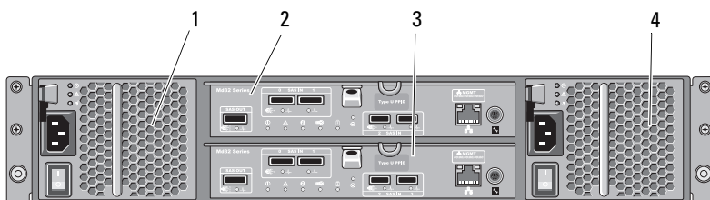
図 2-4. 背面パネルの機能およびインジケータ —Dell PowerVault MD3200 シリーズ
