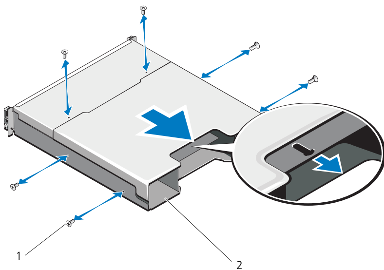
図 15-15. RAID コントローラモジュール / 電源装置ケーシングの取り外しと取り付け
