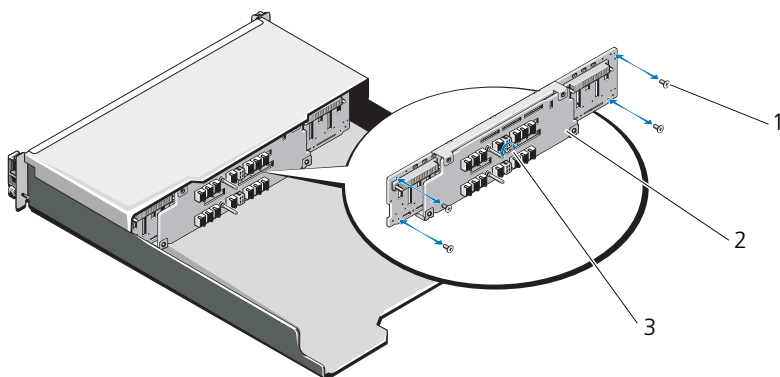
図 15-17. バックプレートの取り外しと取り付け — PowerVault MD3220
