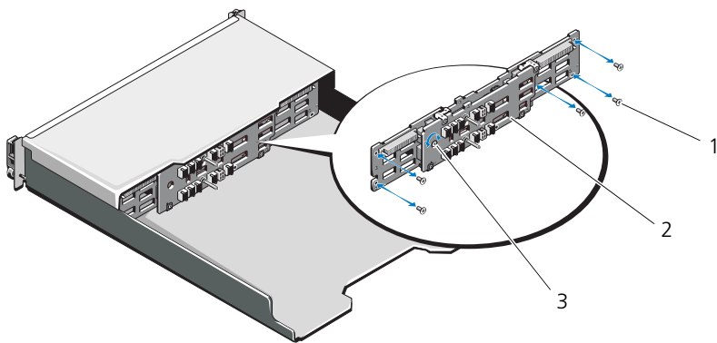
図 15-16. バックプレートの取り外しと取り付け — PowerVault MD3200
