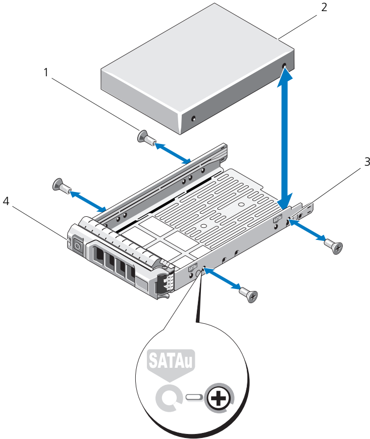
図 15-5. 3.5 インチハードディスクドライブキャリアでのハードディスクドライブの取り外しおよび取り付け
