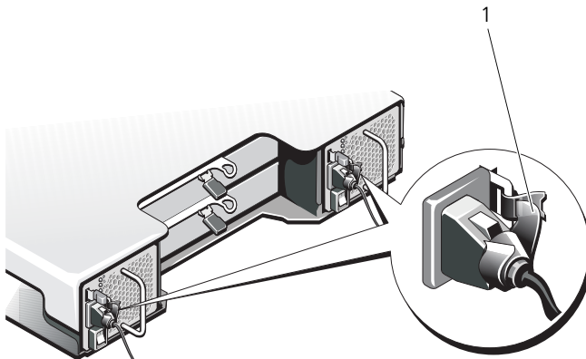
図 15-12. 電源ケーブルの固定
