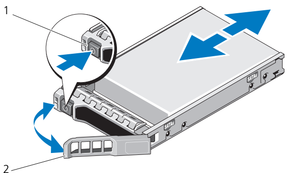
図 15-4. ハードディスクドライブの取り外しと取り付け
