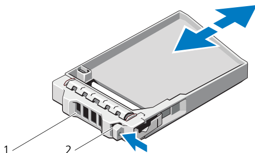
図 15-3. 2.5 インチハードディスクドライブダミーの取り外しおよび取り付け (MD3220 のみ)
