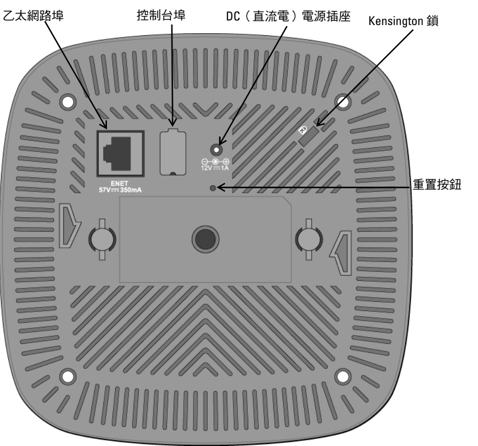
圖2 W-AP103 後視圖
