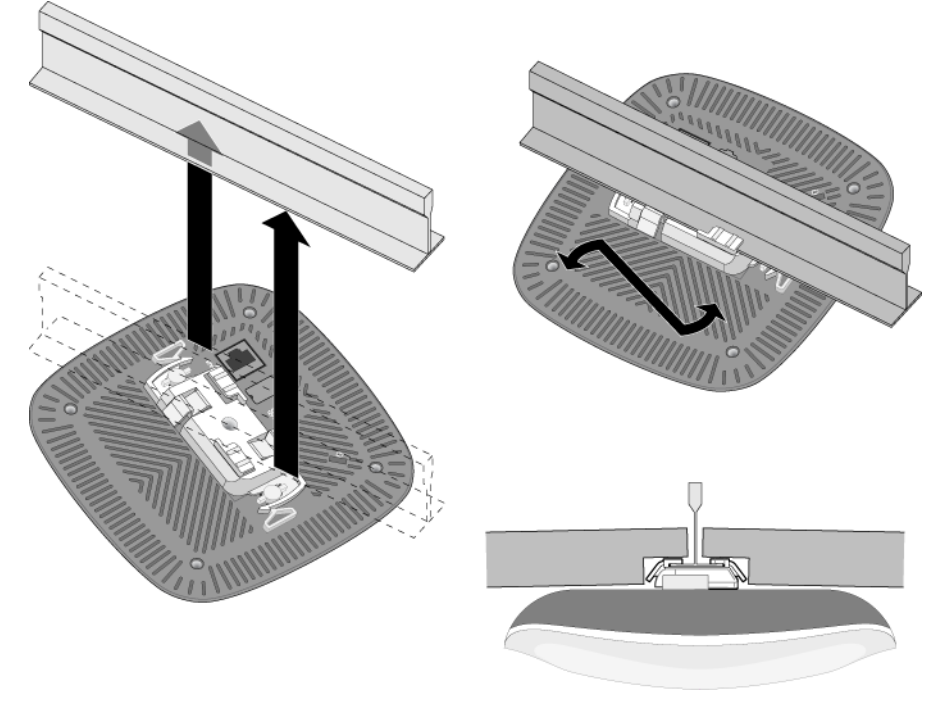
圖 5 安裝 AP
