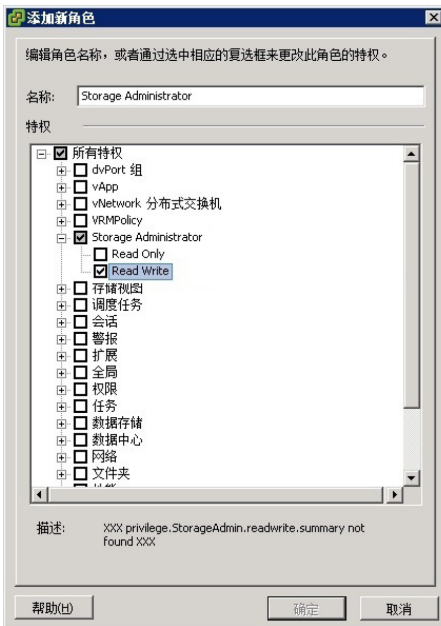
图 4: 添加新角色
