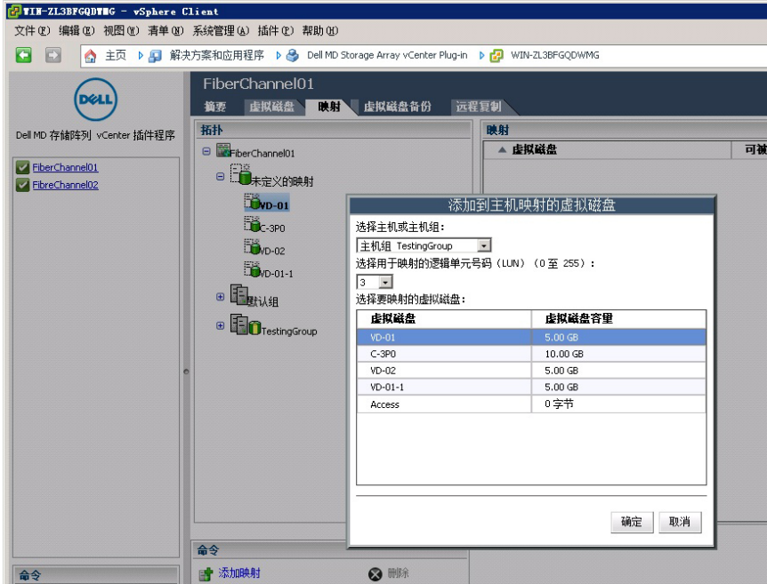
图 47: 虚拟磁盘映射视图
