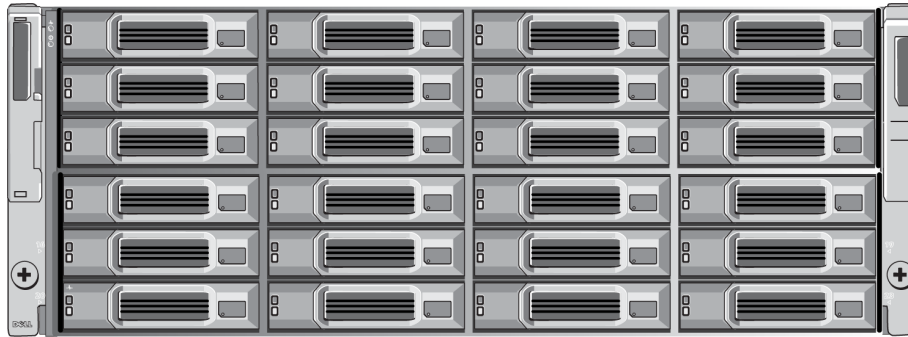
図 3: 4U アレイ - 前面図(ベゼルなし)
