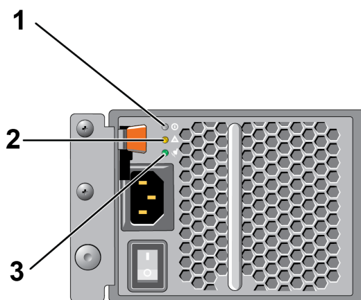
図 9: AC 電源装置スイッチと LED(2U アレイ)
