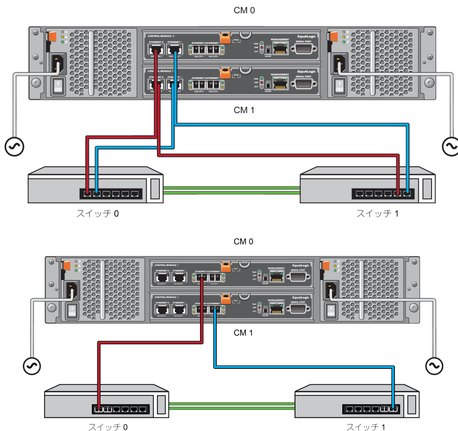
図 6: 推奨ネットワーク構成
