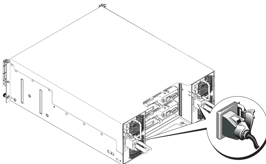
図 8: AC 電源ケーブルの接続(4U アレイ)
