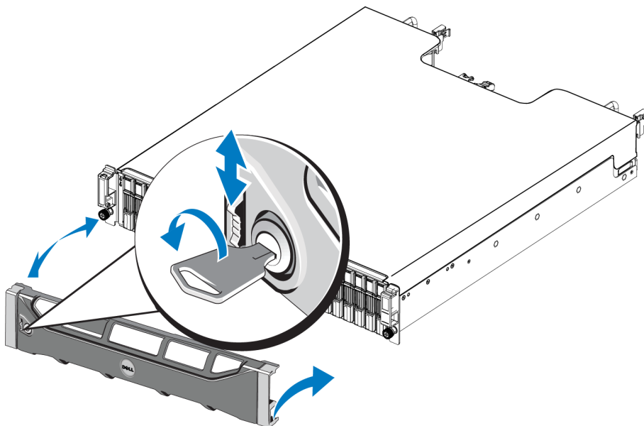
図 4: ベゼルの取り付け(2U アレイ)
