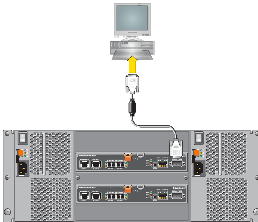
図 11: シリアルケーブルのアレイへの接続 (4U アレイ)
