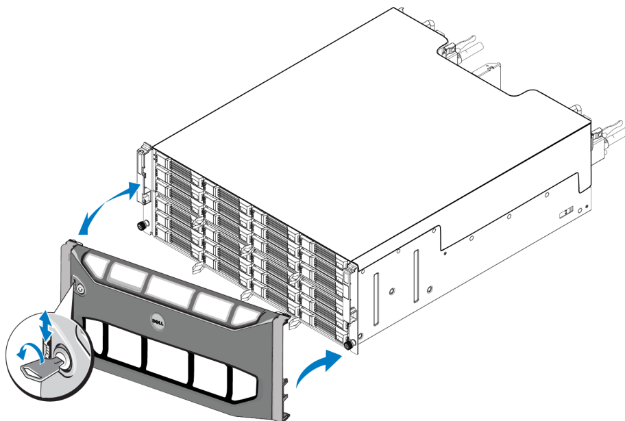
図 5: ベゼルの取り付け(4U アレイ)
