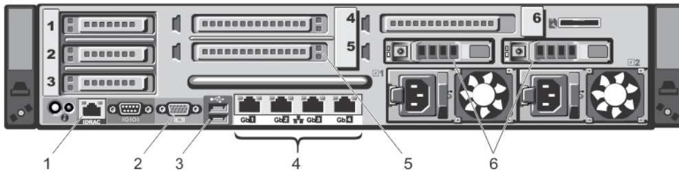
그림 7 . DR4100 System Rear Chassis Port Locations
