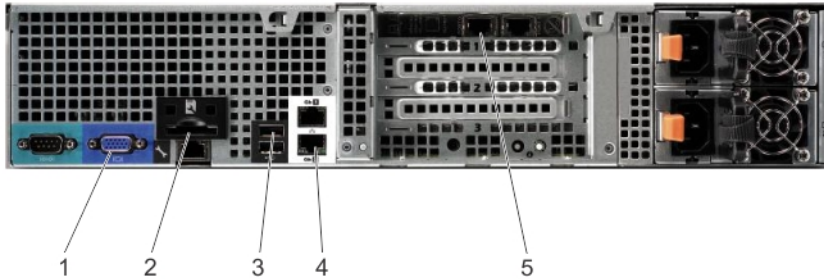
그림 6 . DR4000 System Rear Chassis Port Locations
