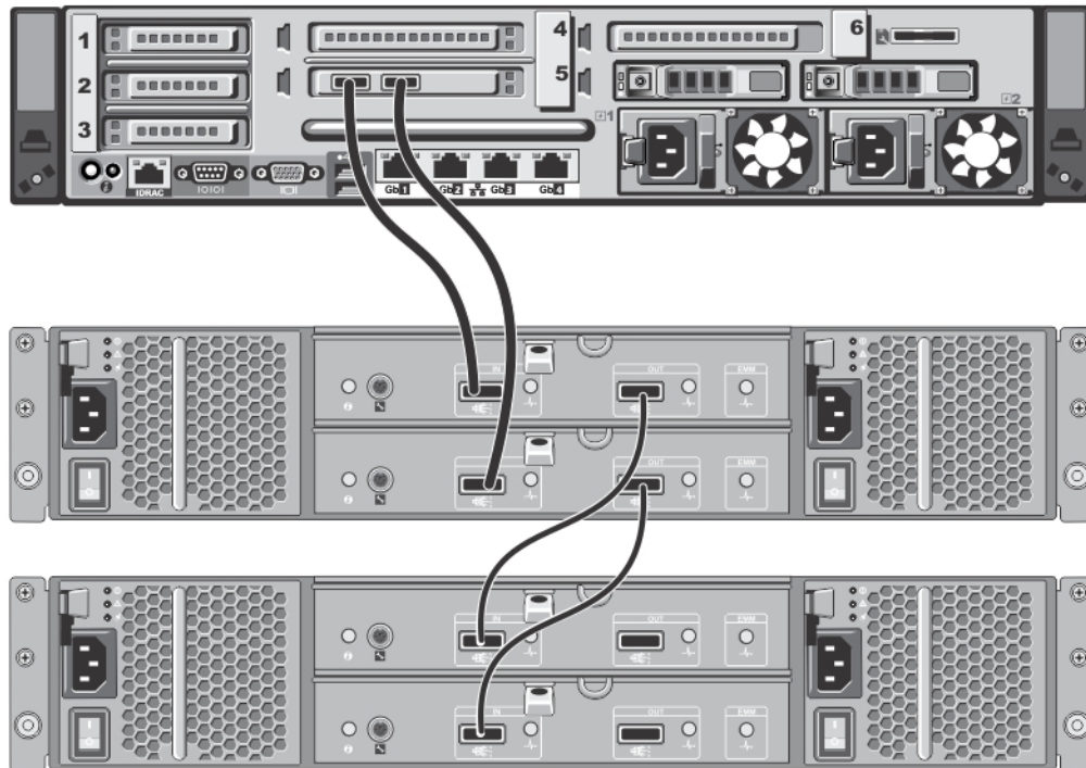
그림 4 . Unified Mode Daisy-Chained Redundant Path Dell PowerVault MD1200 Enclosures
