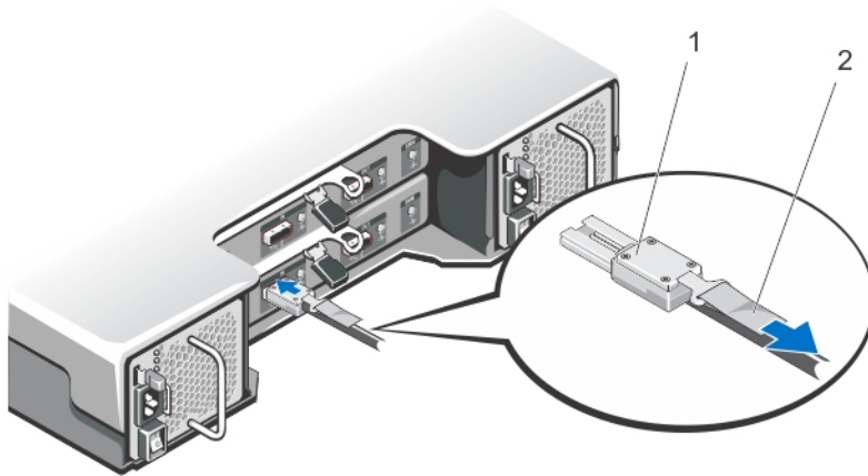
그림 5. SAS Port and Cable Connections (Dell PowerVault MD1200 EMM)
