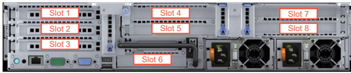
■ 8 x PCIe スロット構成
