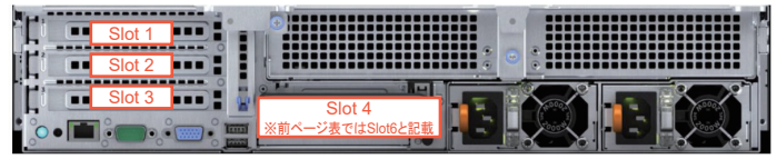
■ 4 x PCIe スロット構成(ダブルワイドスロットなし)
