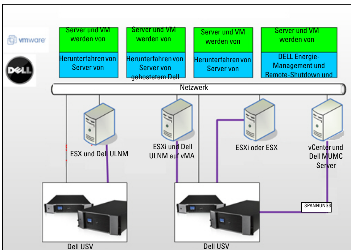
Abbildung 61. Dell ULNM- und Dell MUMC-Konfigurationen für VMware
