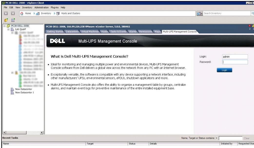
Abbildung 95. vCenter Server-Konsole
