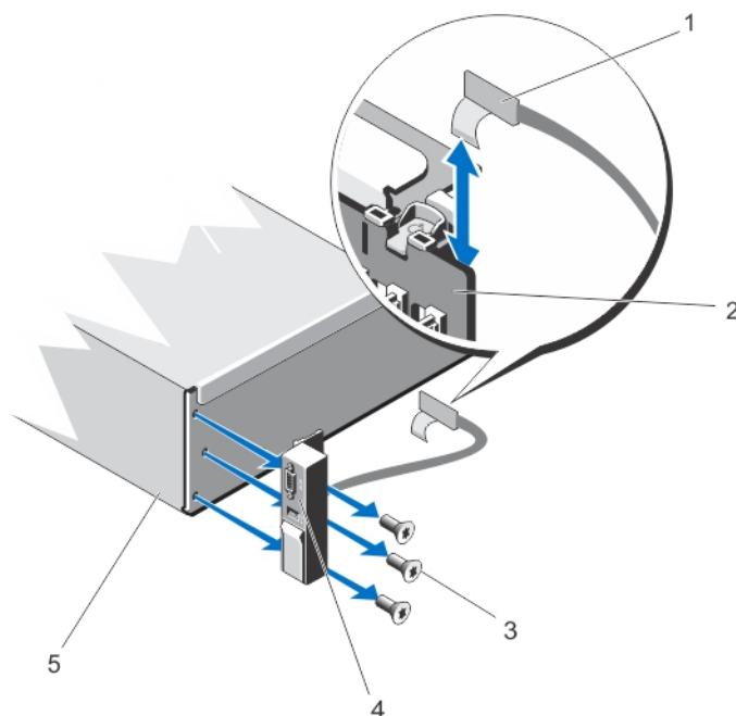
Figure 44. Retrait et installation du panneau d'E/S
