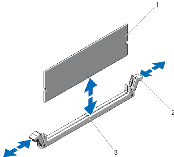
Figure 12. Retrait et installation d'une barrette de mémoire
