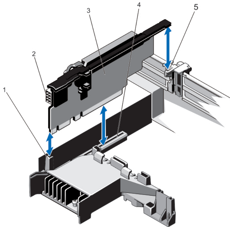
Figure 28. Retrait et installation de la carte de montage de carte d'extension 3
