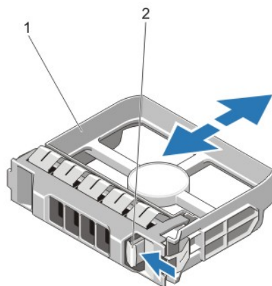
Figure 13. Retrait et installation d'un cache de disque dur de 3,5 pouces
