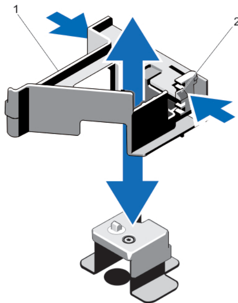
Figure 19. Retrait et installation du support carte PCIe
