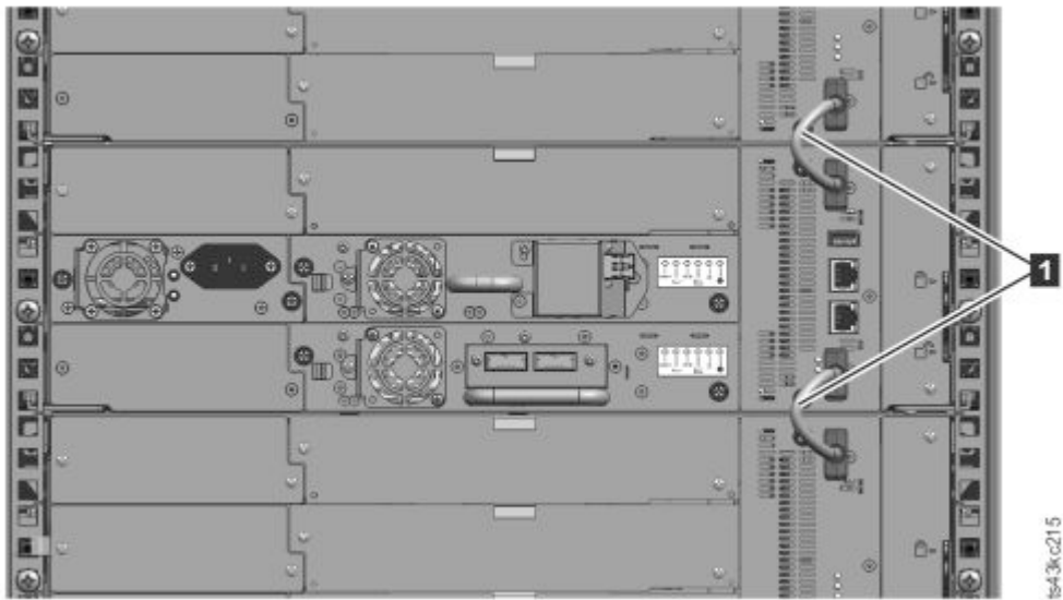
그림 48. 연결된 모듈
