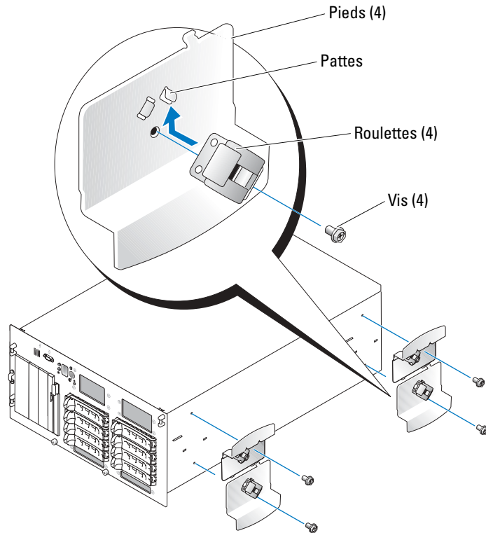
Figure 1. Fixation de roulettes sur le système
