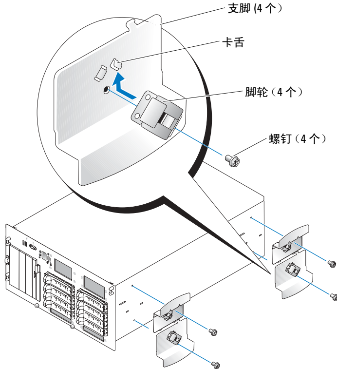
图 1. 在系统上安装脚轮
