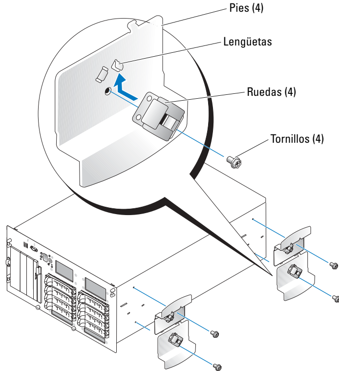
Figura 1. Fijación de las ruedas al sistema
