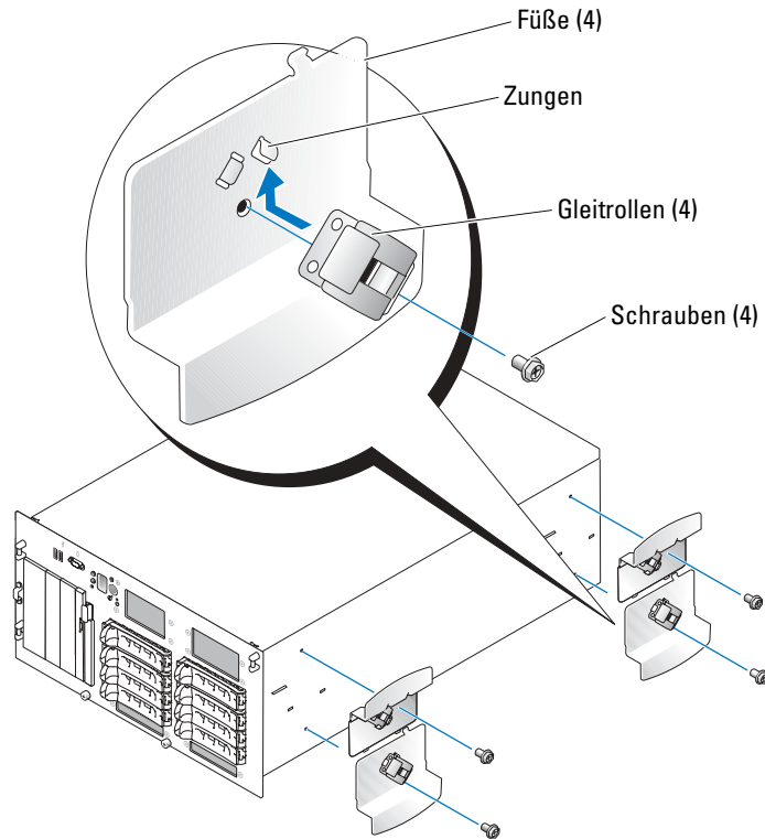
Abbildung 1. Montieren von Gleitrollen an das System
