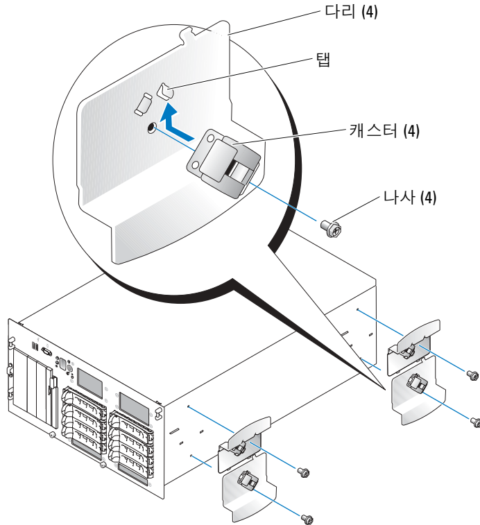
그림 1. 캐스터를 시스템에 연결
