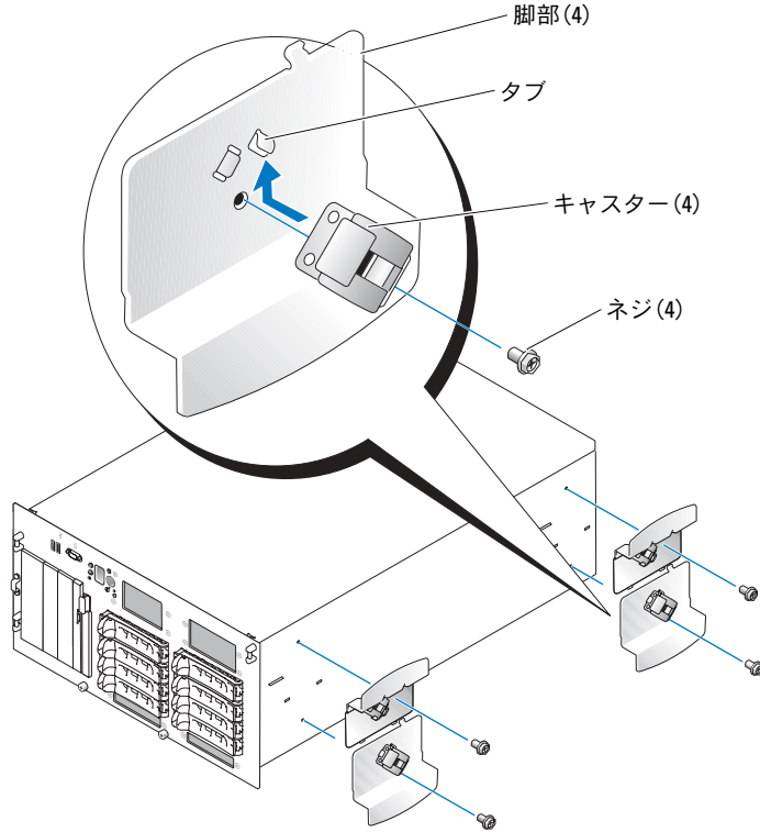
図 1. システムへのキャスターの取り付け
