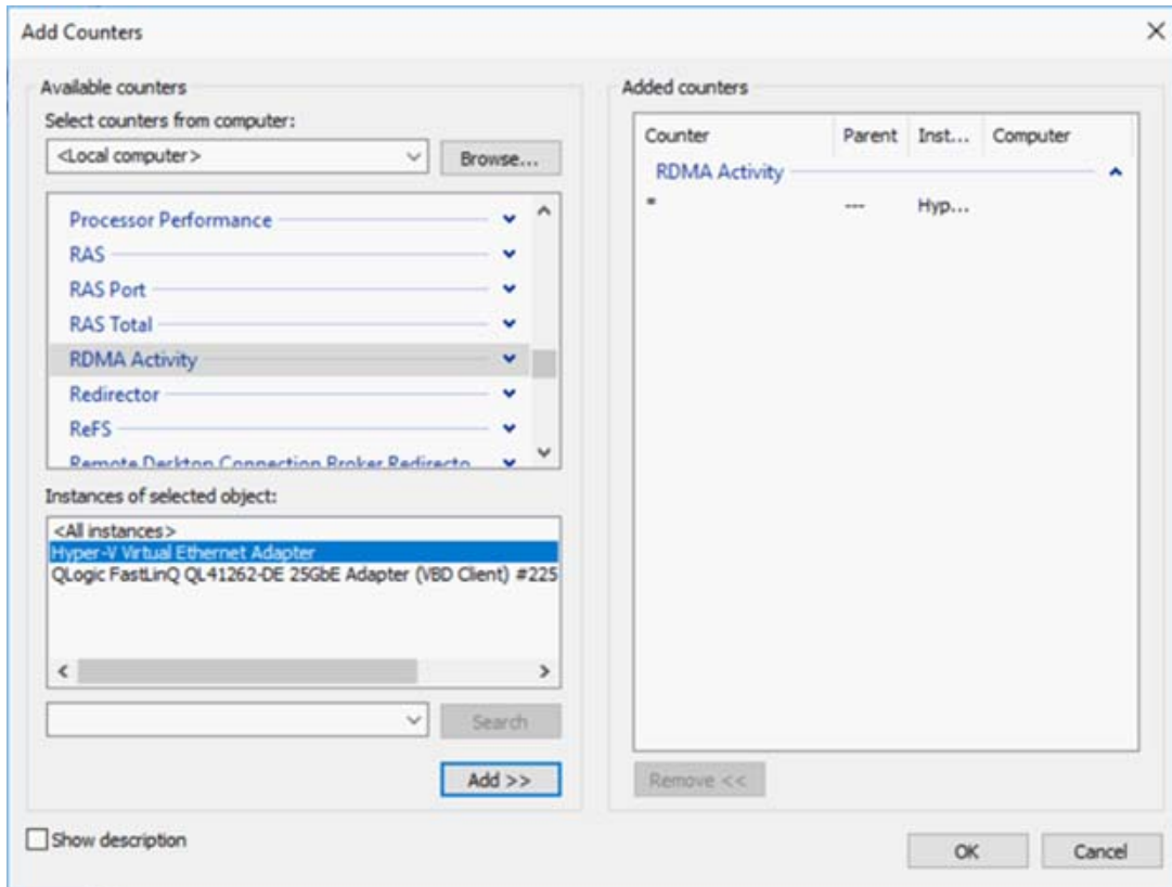
図 13-5. カウンタの追加ダイアログボックス
