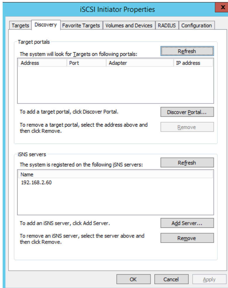
図 9-19. iSCSI イニシエータ — ターゲットポータルの検出
