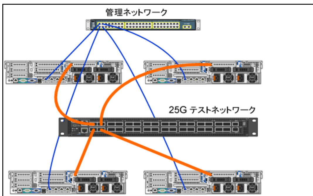
図 13-18. ハードウェア構成の例
