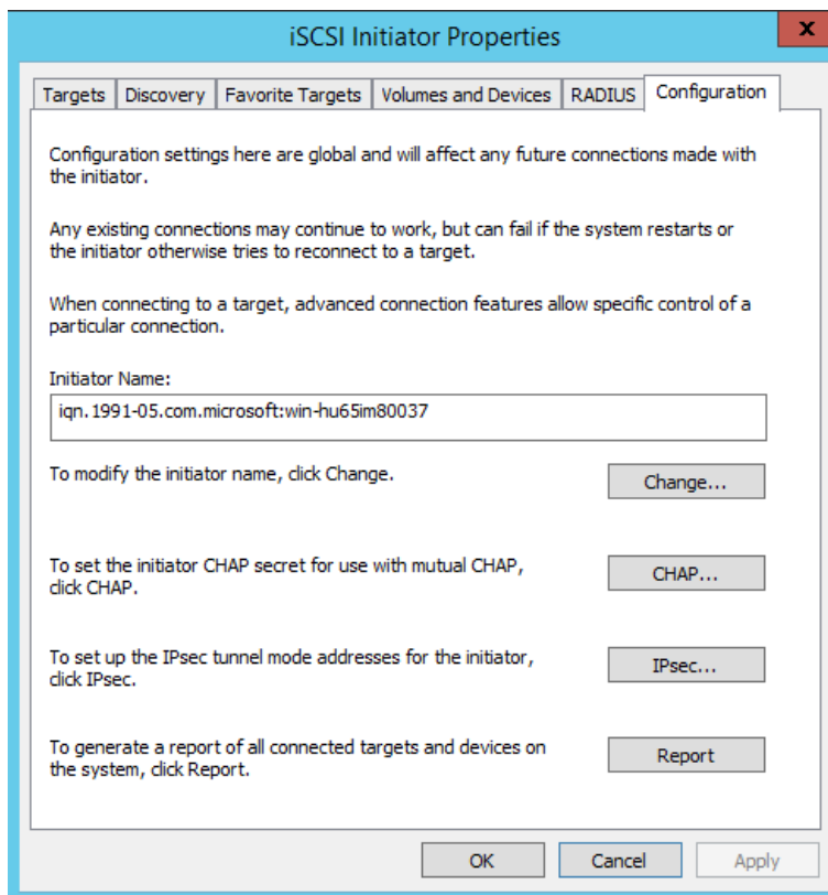
図 9-17. iSCSI イニシエータプロパティ、設定ページ
