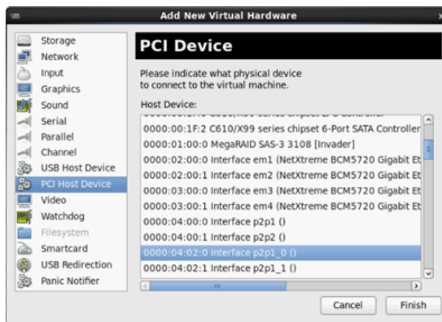
図 11-14. 新しい仮想ハードウェアの追加
