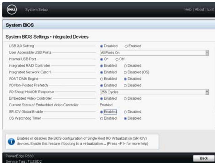
図 11-1. SR-IOV のセットアップユーティリティ：統合デバイス
