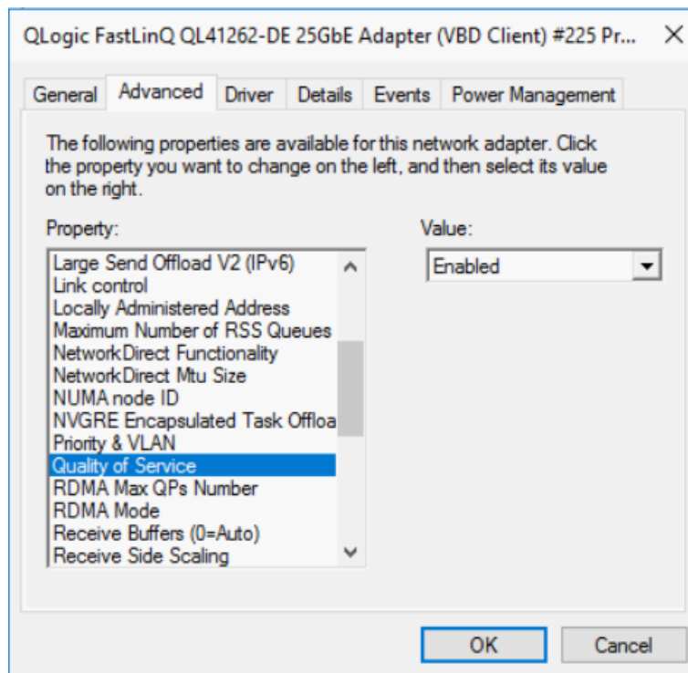
図 13-11. 詳細設定プロパティ : QoS の有効化
