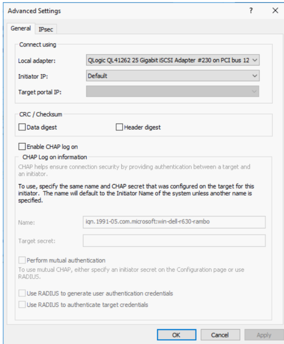
図 9-21. Initiator IP アドレスの選択
