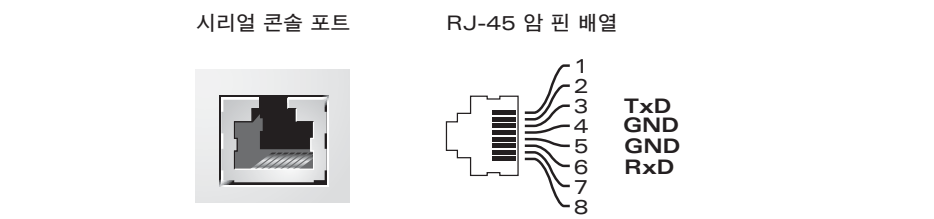
그림 4 시리얼 포트 핀 배열
