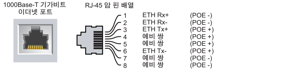
그림 5 기가비트 이더넷 포트 핀 배열
