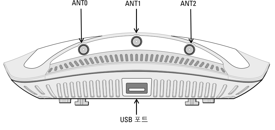
그림 2 W-AP110 시리즈 측면 보기(W-AP114 표시)
