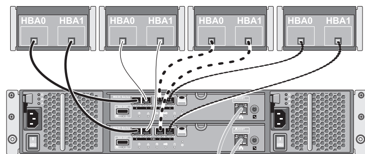
图 2-5. 使用电缆将一个四节点直接连接的群集连接至 PowerVault MD36x0f 存储系统
