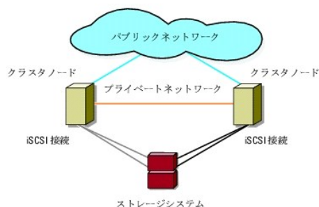
図 2-4 直接接続のクラスタ構成
