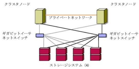
図2-13 4 台のストレージシステムにケーブル接続された PowerEdge クラスタノード
