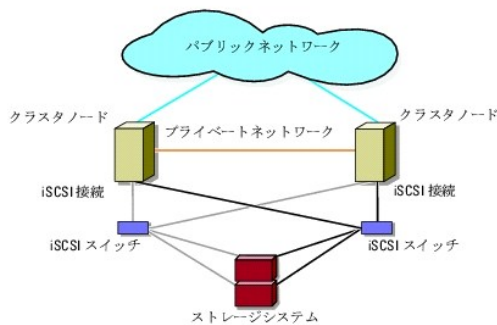
図 2-9 iSCSI スイッチ接続の 8 ノードクラスタ
