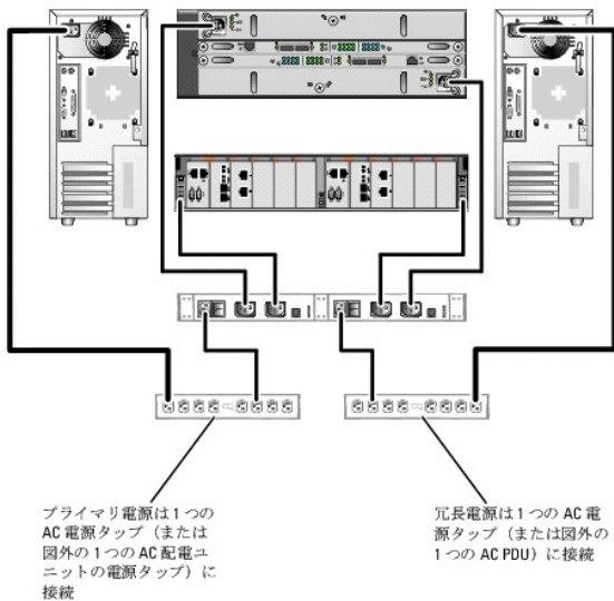
図 2-1 1 台の電源ユニットを使用した PowerEdge システムの電源ケーブル接続の例
