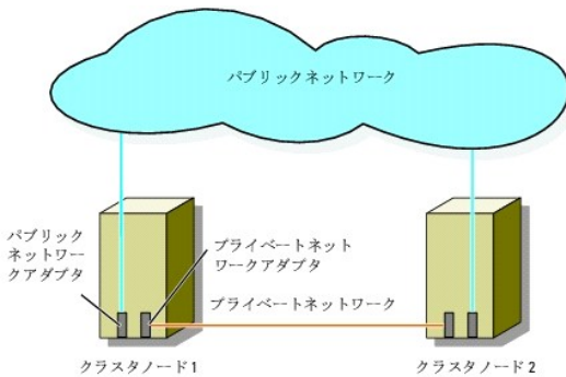
図 2-3 ネットワークのケーブル接続の例
