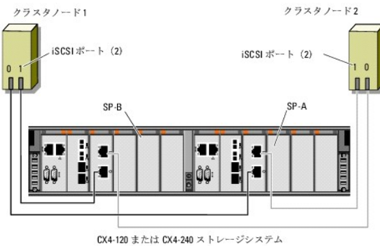
図 2-6 2 ノードのクラスタから CX4-480 ストレージシステムへのケーブル接続
