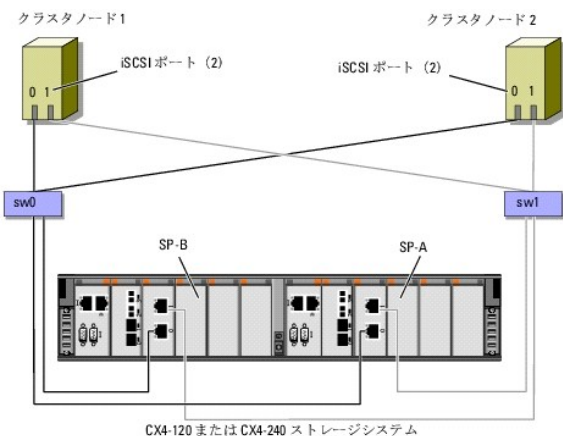
図2-11 1 つの iSCSI 接続クラスタから Dell/EMC CX4-480 へのケーブル接続
