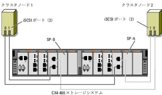
図 2-7 2 ノードのクラスタから CX4-960 ストレージシステムへのケーブル接続
