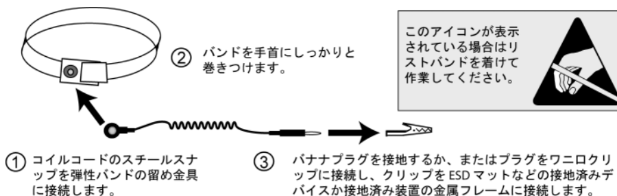
図 1-4: 静電気防止用リストバンドの使用
