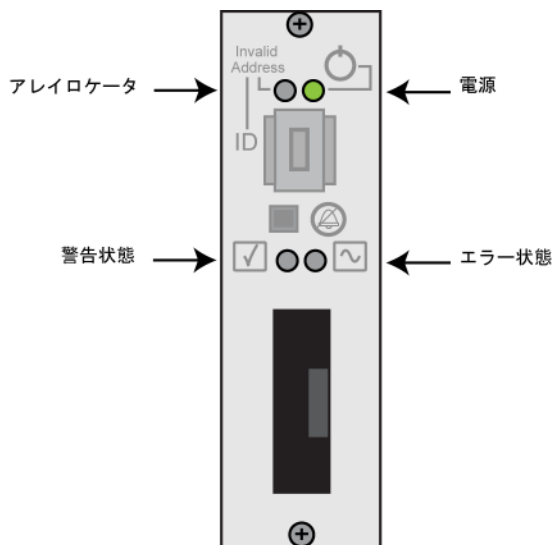
図 1-3: 操作パネルの LED
