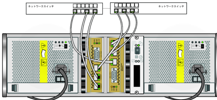
図 3-4: 推奨されるデュアルコントロールモジュールの構成
