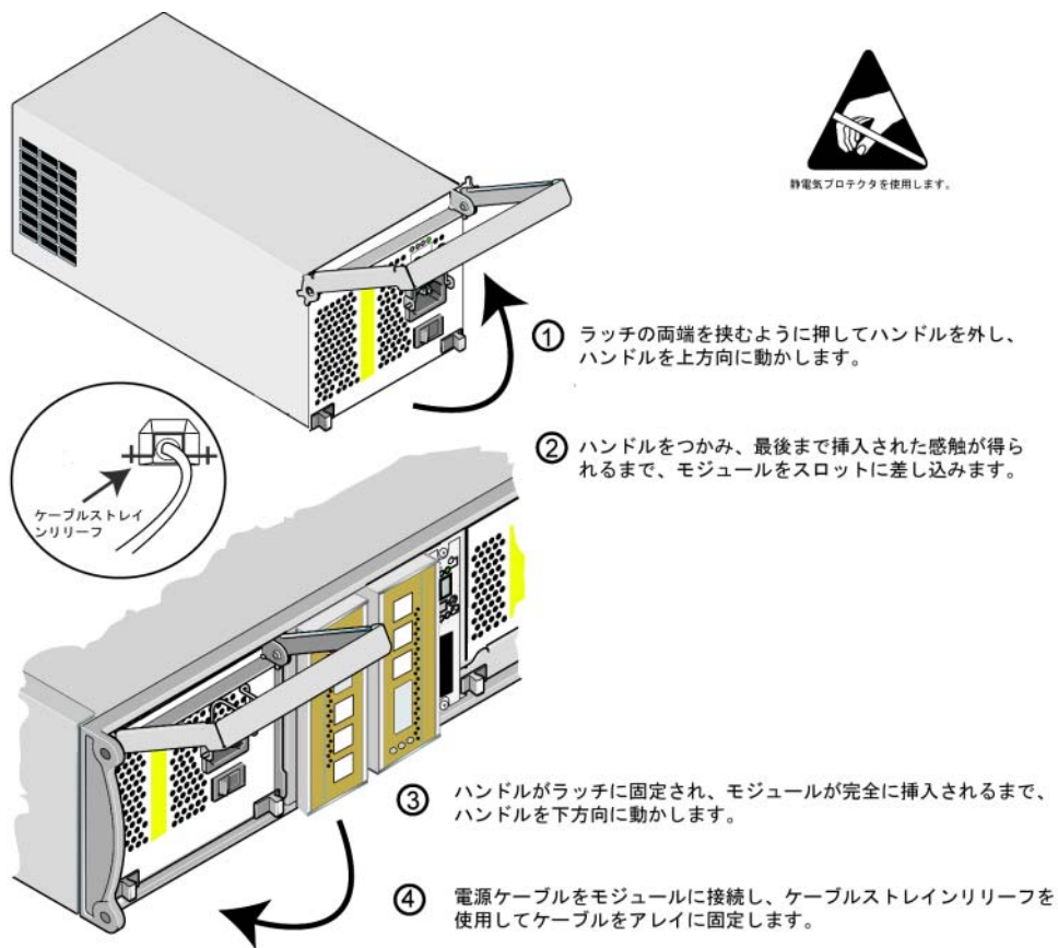
図 4-3: PSU/ 冷却モジュールの取り付け
