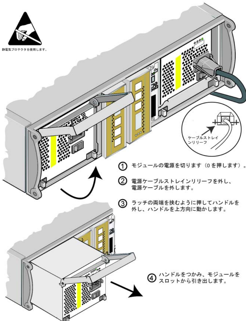
図 4-2: PSU/ 冷却モジュールの取り外し
