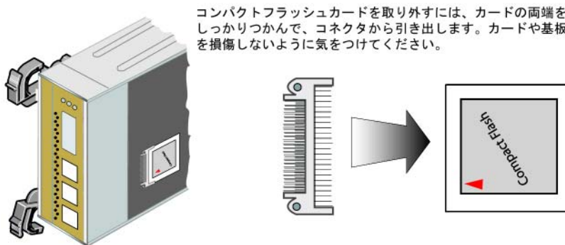
図 3-7: コンパクトフラッシュカードの取り外しと取り付け
