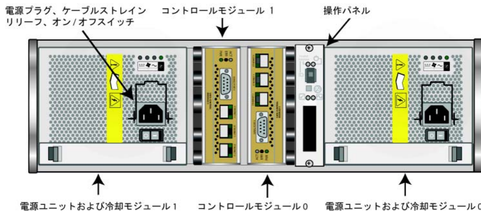
図 1-2:PS5000 背面パネル
