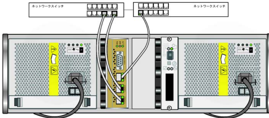
図 3-2: 推奨されるシングルコントロールモジュールの構成
