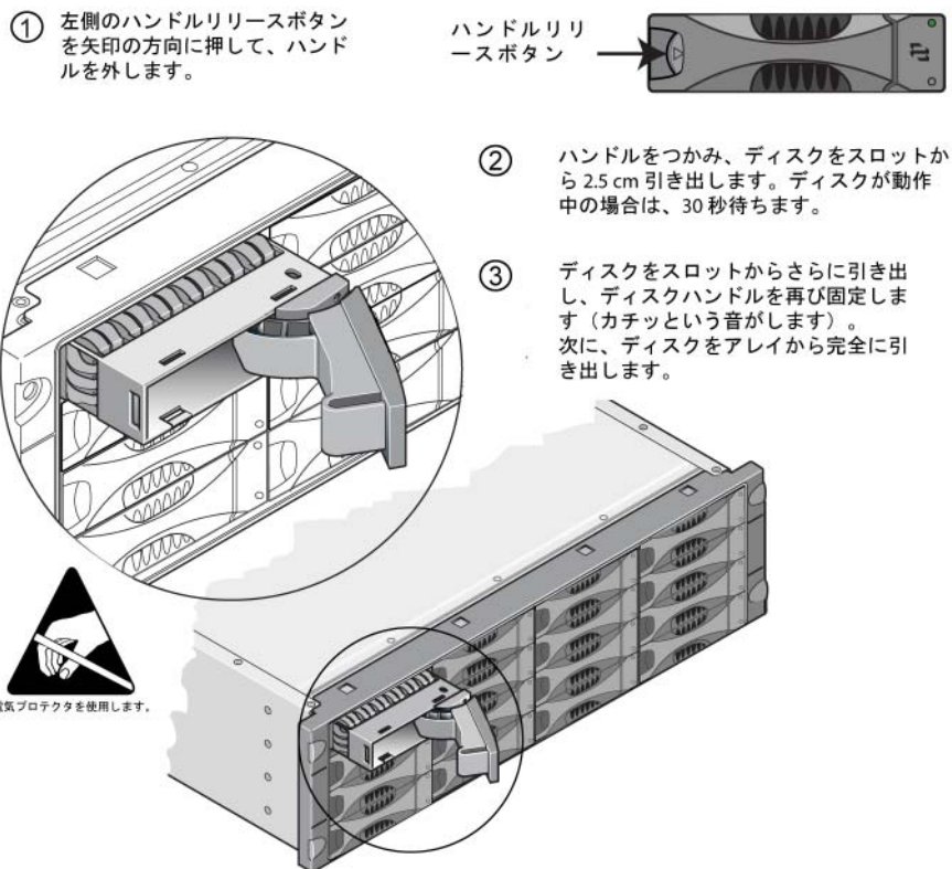
図 2-3: ディスクの取り外し
