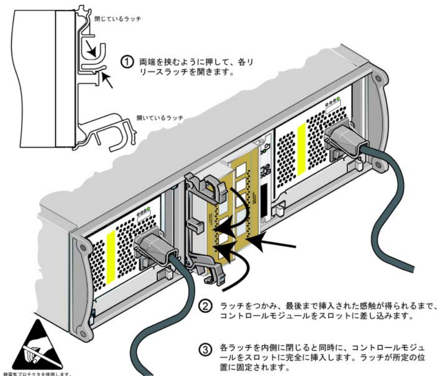
図 3-6: コントロールモジュールの取り付け
