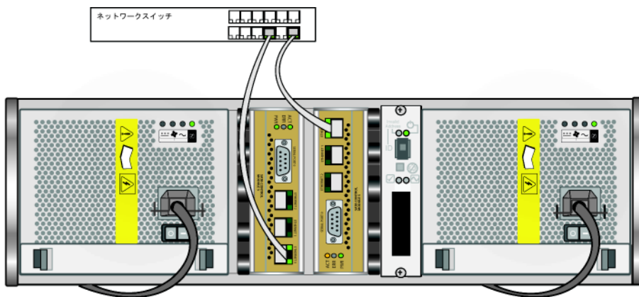
図 3-3: 最小限必要なデュアルコントロールモジュールの構成
