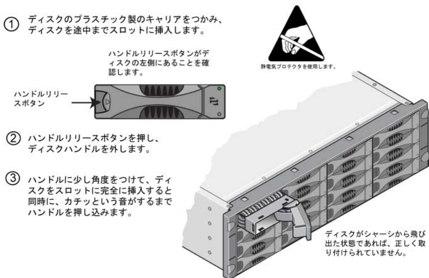
図 2-4: ディスクの取り付け
