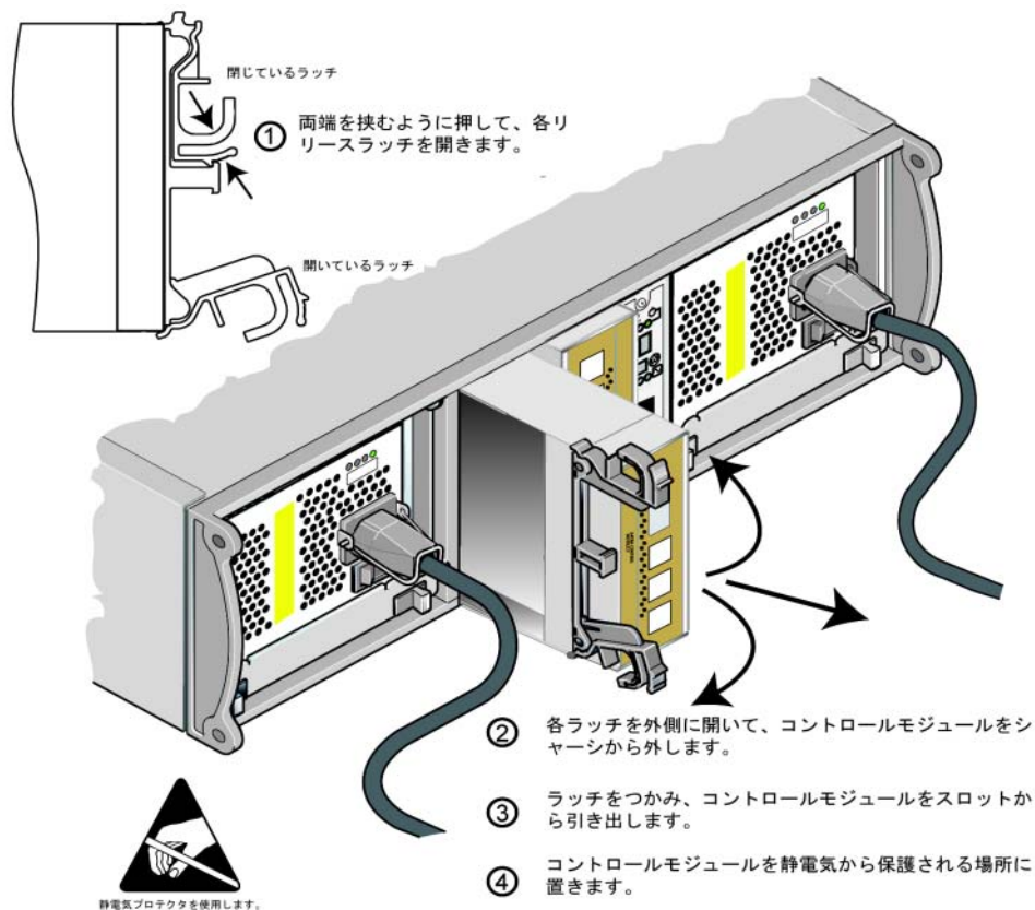
図 3-5: コントロールモジュールの取り外し
