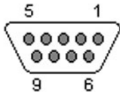
图 10: 串行电缆 DB9 连接器 - 插针位置
