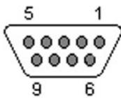
Ilustración 10. Conector DB9 de cable serie: Ubicaciones de las patas
