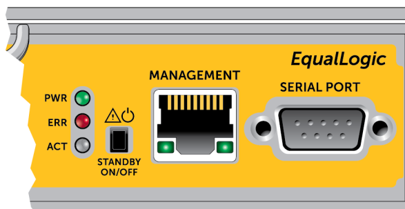
図 22: 管理ポートの位置
