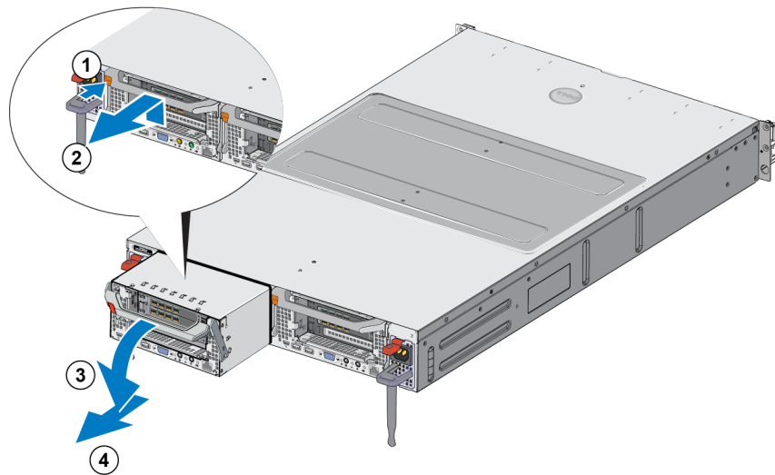
Figure 7 : Retrait d'un contrôleur
