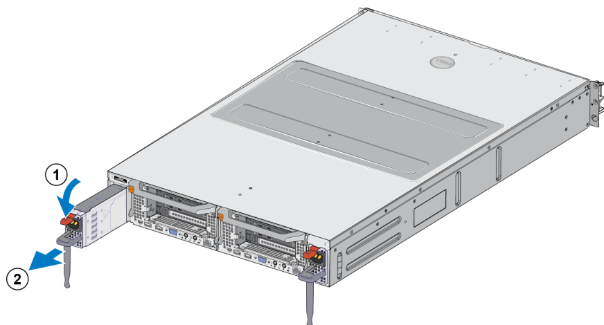
Figure 9 : Retrait d'un bloc d'alimentation
