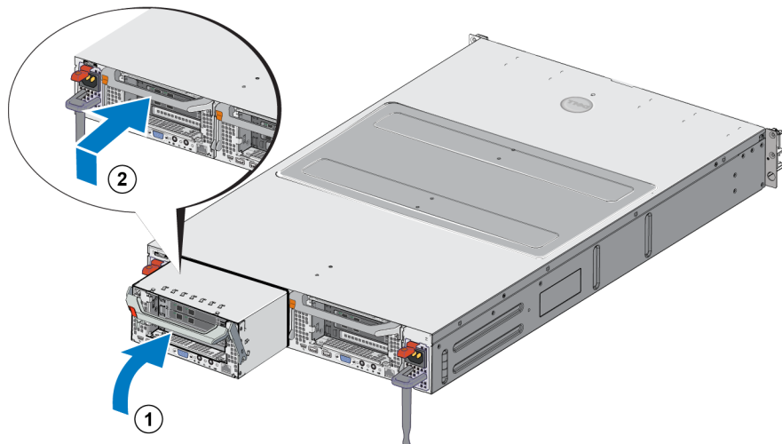
Figure 8 : Installation d'un contrôleur
