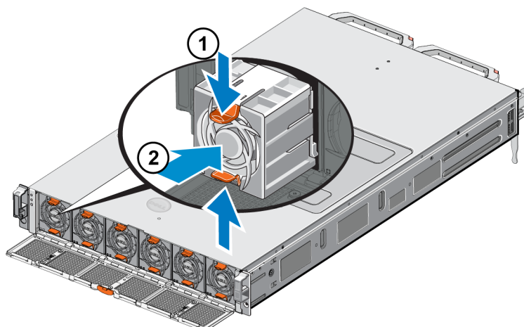
Figure 15 : Installation d'un ventilateur de refroidissement
