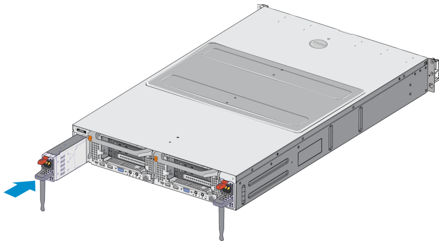
Figure 10 : Installation d'un bloc d'alimentation
