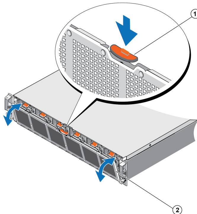
Figure 13 : Ouverture et fermeture du capot d'accès au ventilateur de refroidissement
