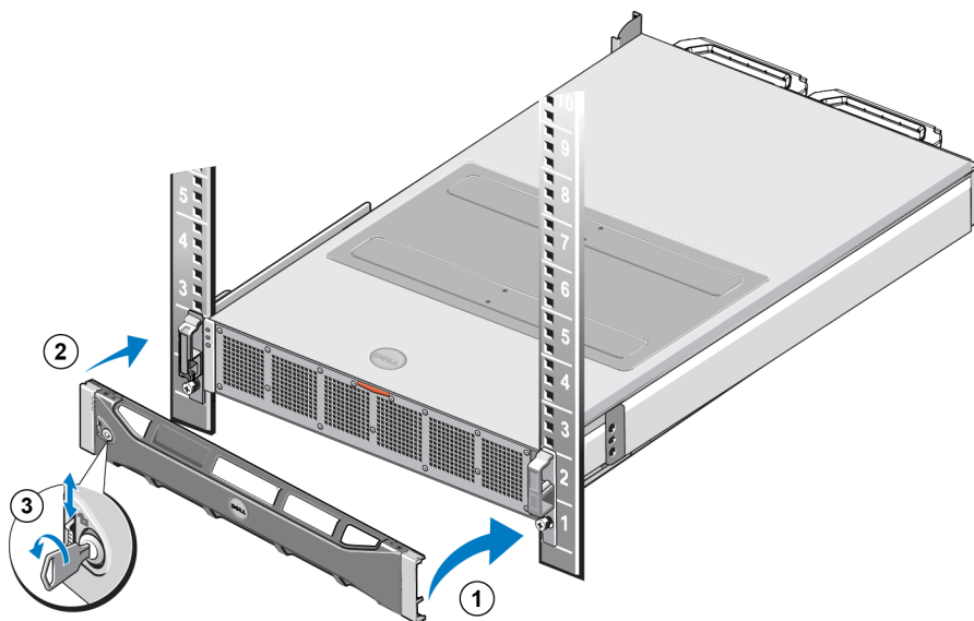
Figure 12 : Fixation du cadre
