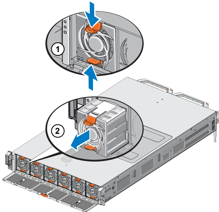
Figure 14 : Retrait d'un ventilateur de refroidissement
