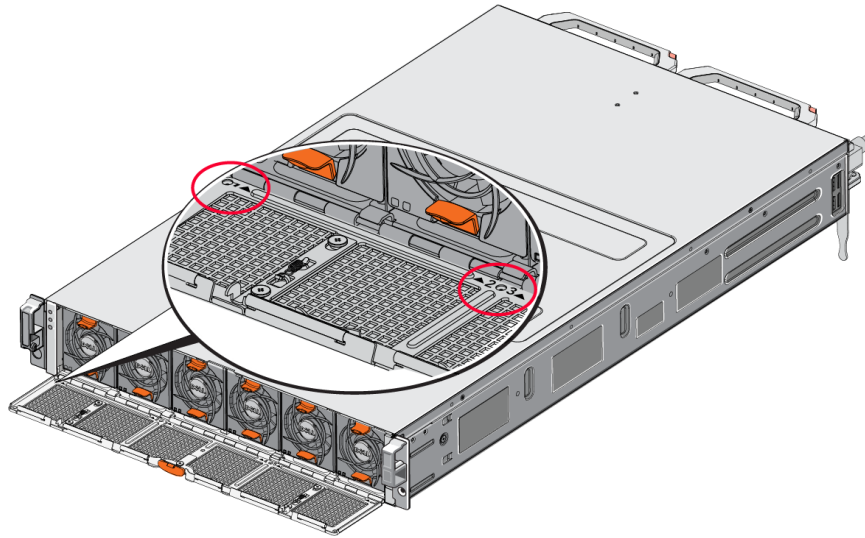
Şekil 2: FS7600 Ön Panel (Kapak Açık)
