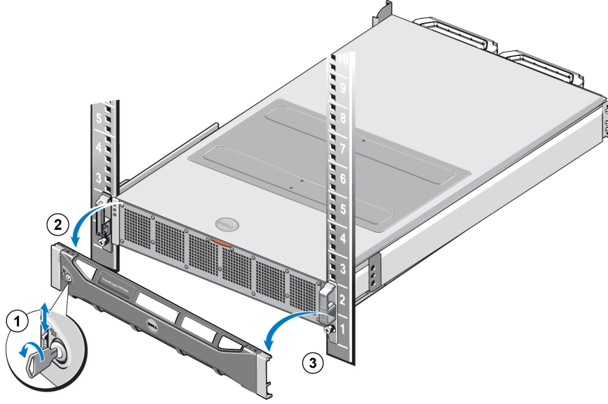
Şekil 11: Çerçevesini Çıkarma
