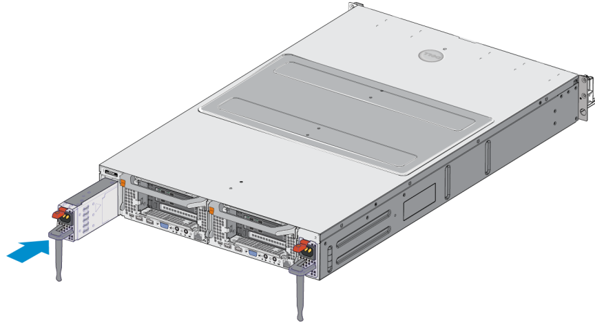
Şekil 10: Güç Kaynağının Takılması
