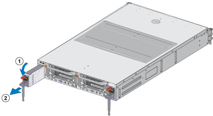
Şekil 9: Güç Kaynağını Çıkarma
