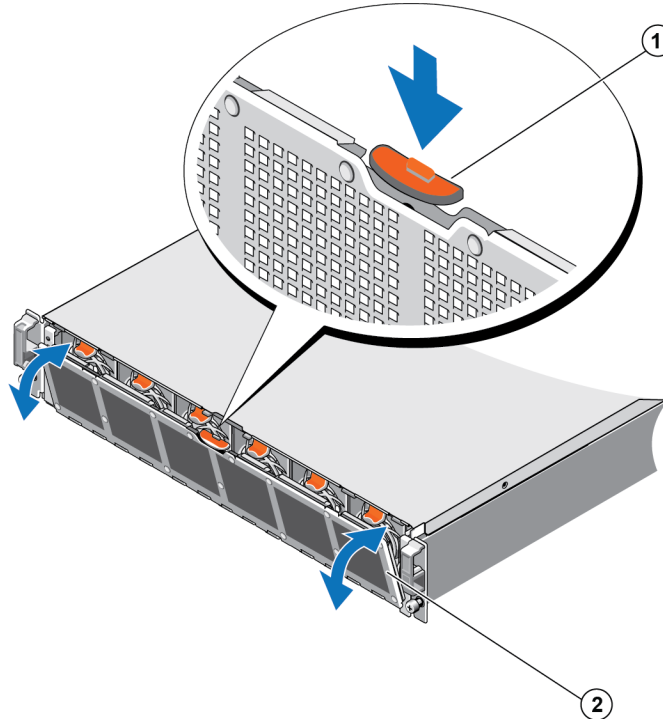
Şekil 13: Soğutma Fanı Erişim Kapağını Açma veya Kapatma
