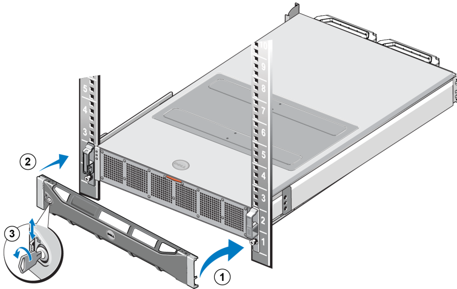
Şekil 12: Çerçeveyi Takma
