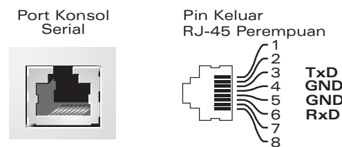
Gambar 4 Pin Keluar Port Serial
