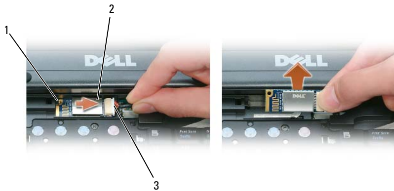
1 Metallklammer 2 Karte 3 Kabelstecker
