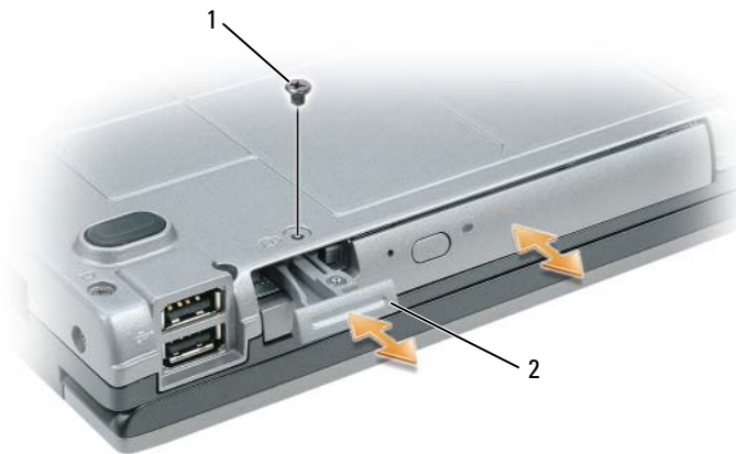
1 Gerätesicherheitsschraube 2 Freigabevorrichtung
