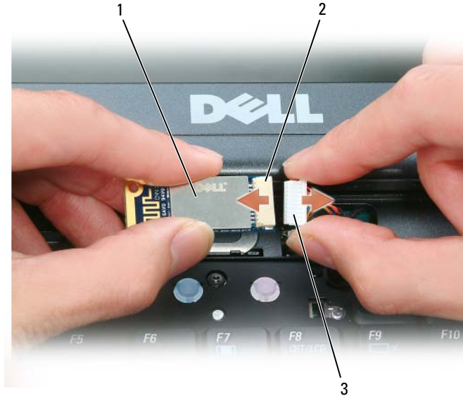
1 Karte 2 Kartenanschluss 3 Kabelstecker
