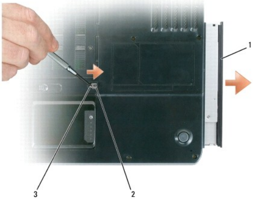
1 光盘驱动器 2 光盘驱动器锁定螺钉 3 槽口
