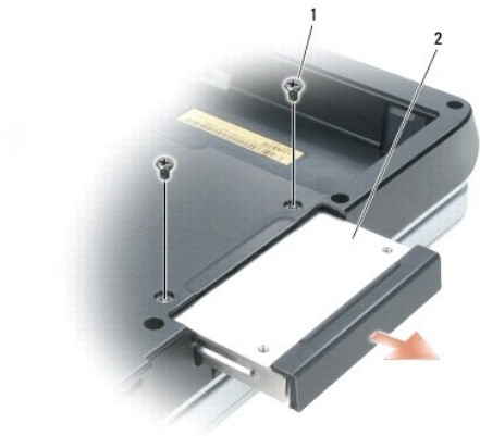
1 螺钉 (2) 2 硬盘驱动器
