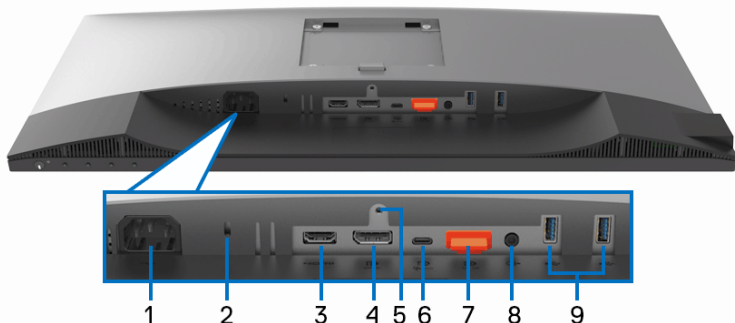
モニタースタンドなし底面図
