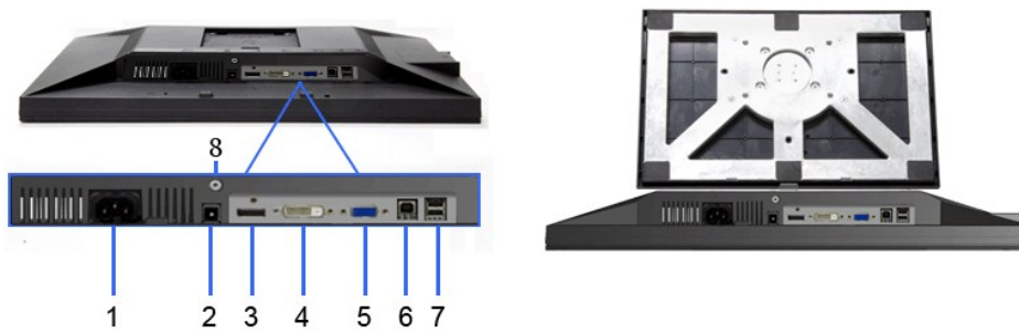
底面図
