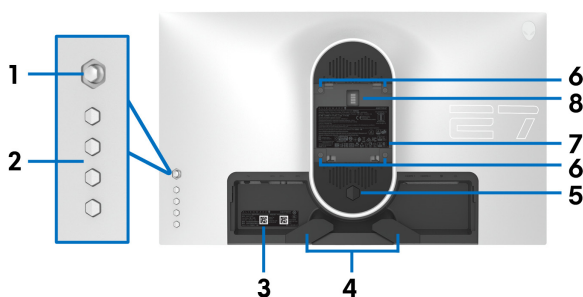
Вид сзади - монитор без стойки
