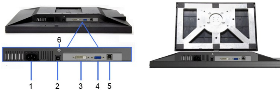
底視圖
