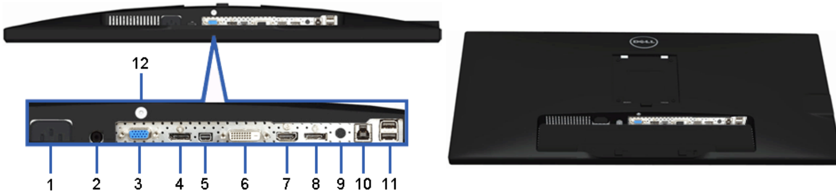
底视图
