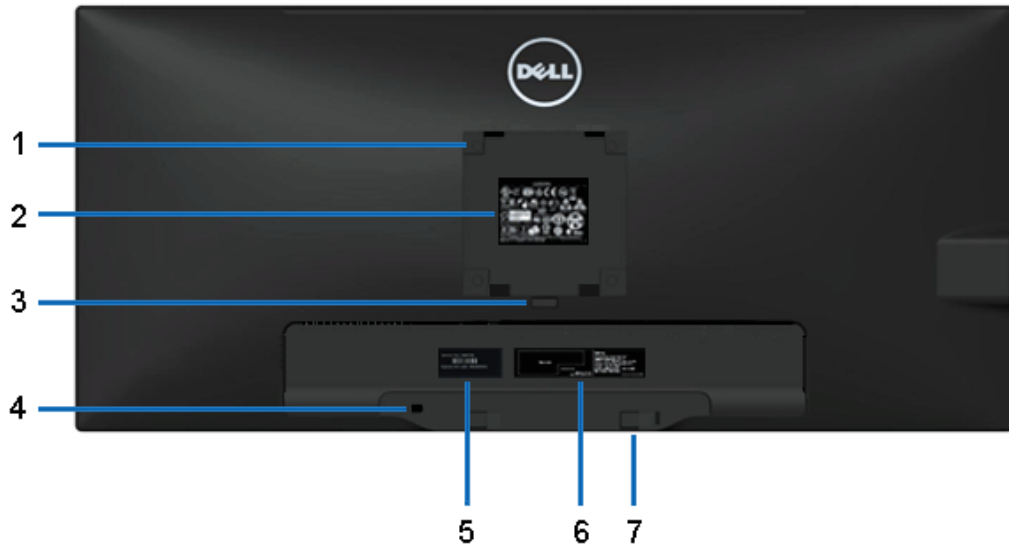
后视图 (包括显示器支架)
