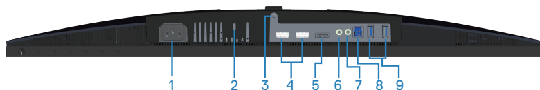
無顯示器立座的底部圖 (S2419HGF)
