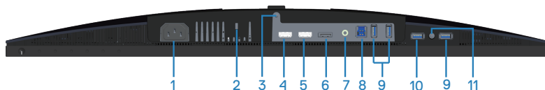
無顯示器立座的底部圖 (S2719DGF)
