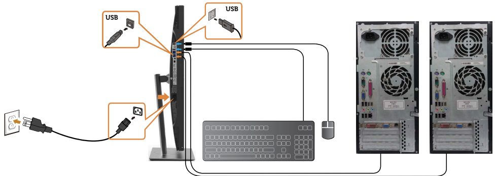
b. Conectar dos ordenadores
