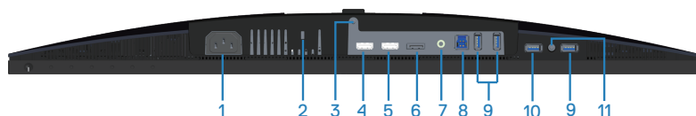
モニタースタンドを取り付けていない状態の底面ビュー（S2719DGF）
