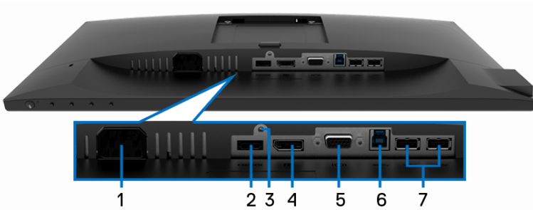
底视图（无显示器支架）
