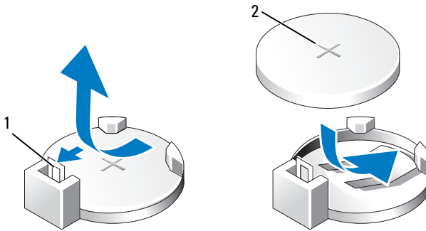
1 Batteriefreigabehebel
