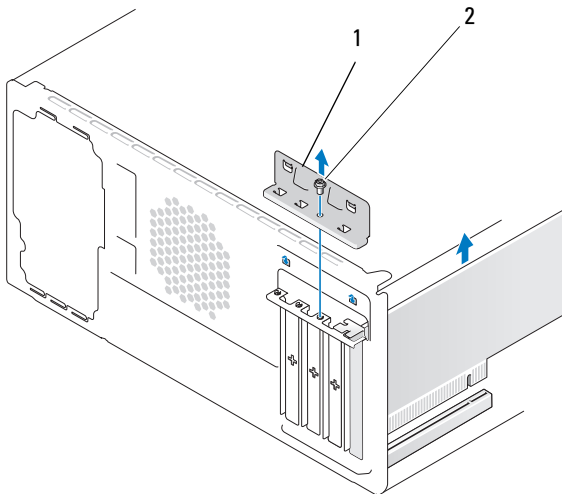
1 kortfastholdelsesbøjle 2 skruer
