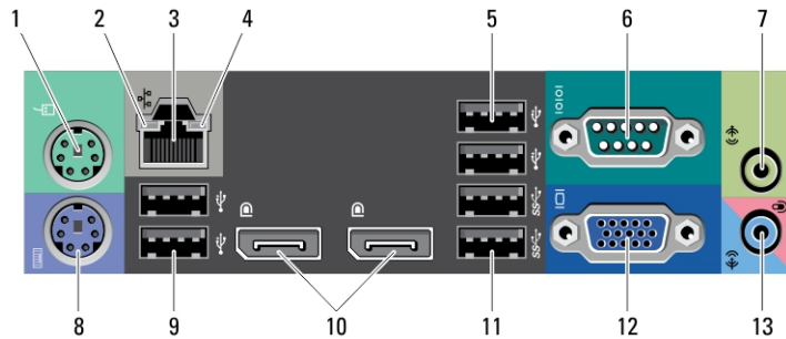
2. ábra. A minitorony hátulnézete
