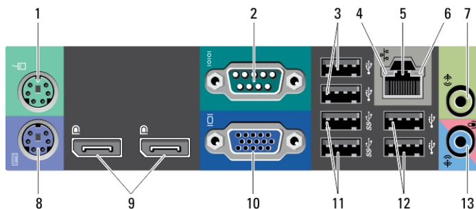
4. ábra. A helytakarékos kivitel hátulnézete
