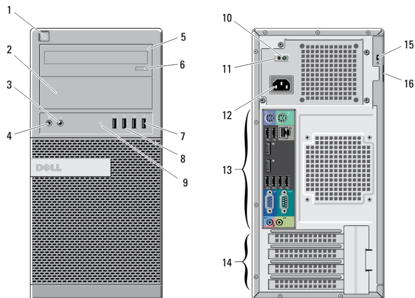
Slika 1. Prikaz kućišta Mini-Tower s prednje i stražnje strane
