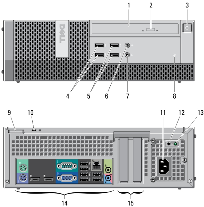
圖 3. 小型電腦的背面板視圖
