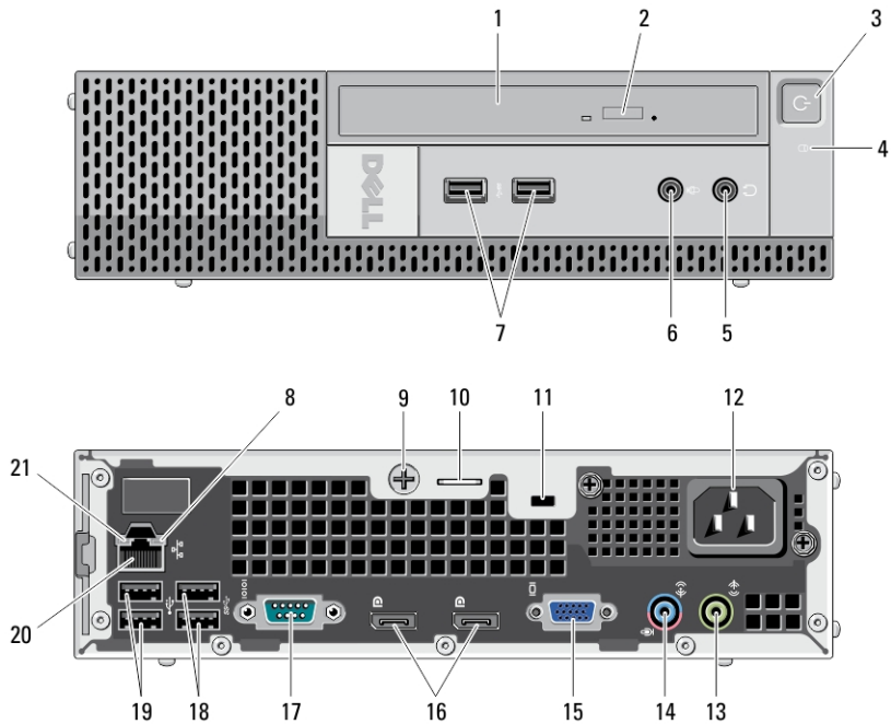
圖 5. 超小型電腦的前視圖與後視圖
