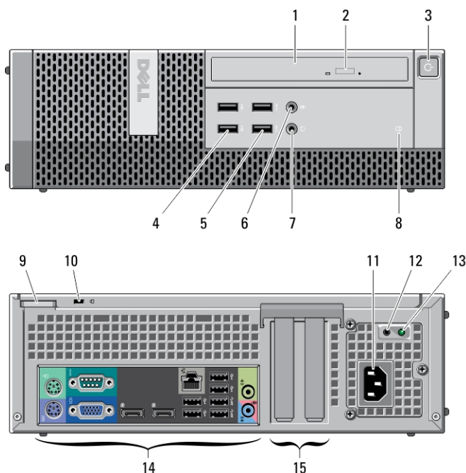
Slika 4. Prednji i stražnji prikaz računala sa SFF kućištem
