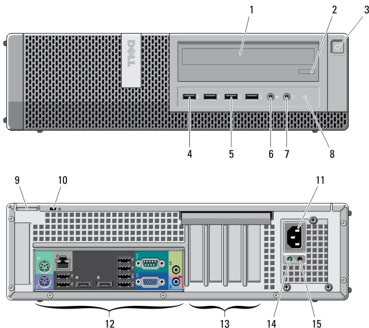
Slika 2. Prikaz stolnog računala s prednje i stražnje strane
