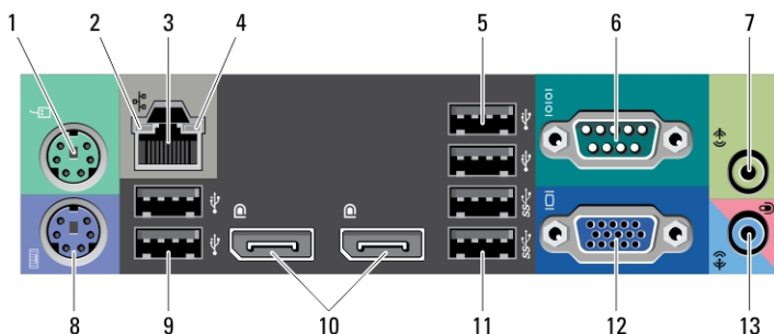
Slika 3. Prikaz stražnje ploče računala s Mini-Tower kućištem i stolnog računala
