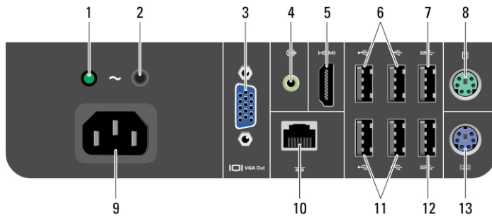
3. ábra. Hátlap nézete
