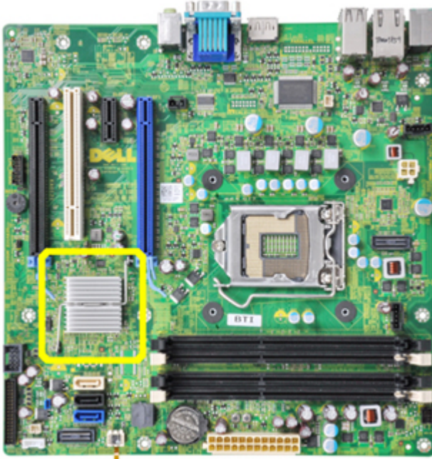
Afbeelding 1. Moederbord van een eerdere versie van het moederbord met de warmteafleider
