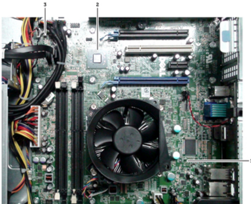
Afbeelding 2. Moederbord zonder warmtesensor en warmteafleider
