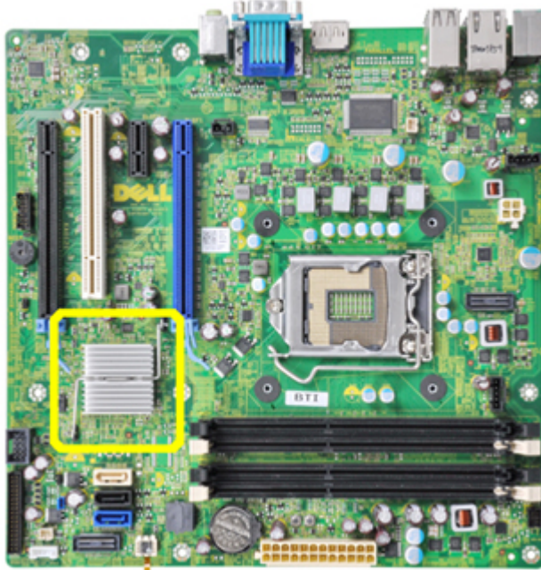
Αριθμός 1. Πλακέτα συστήματος προγενέστερης έκδοσης μαζί με την ψύκτρα
