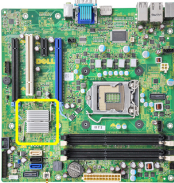
圖 1. 配備散熱器的舊型主機板
