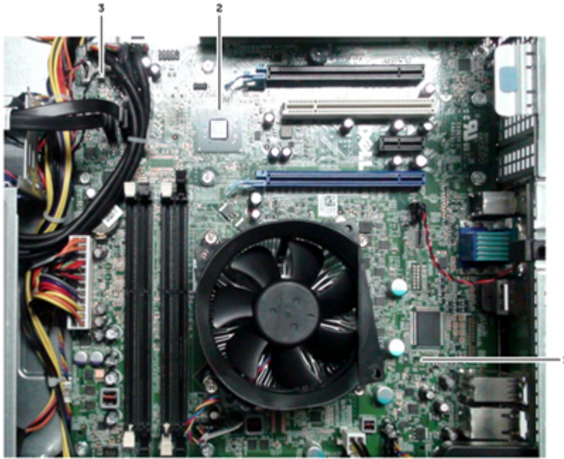
圖 2. 卸下配備熱感應器和散熱器的主機板
