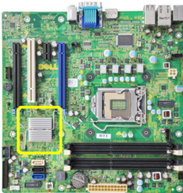
Рисунок 1. Более ранняя версия системной платы с радиатором
