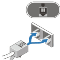
Obrázok 14. Pripojenie modemom
