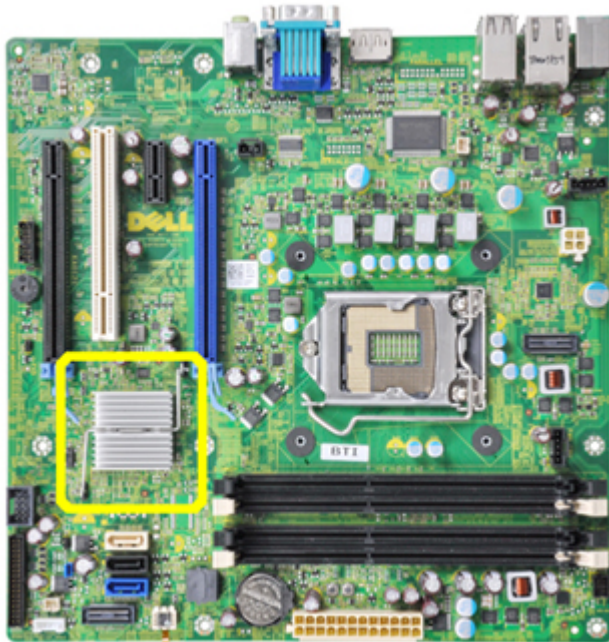
Figura 1. Placa de sistem a unei versiuni anterioare a plăcii de sistem cu radiator
