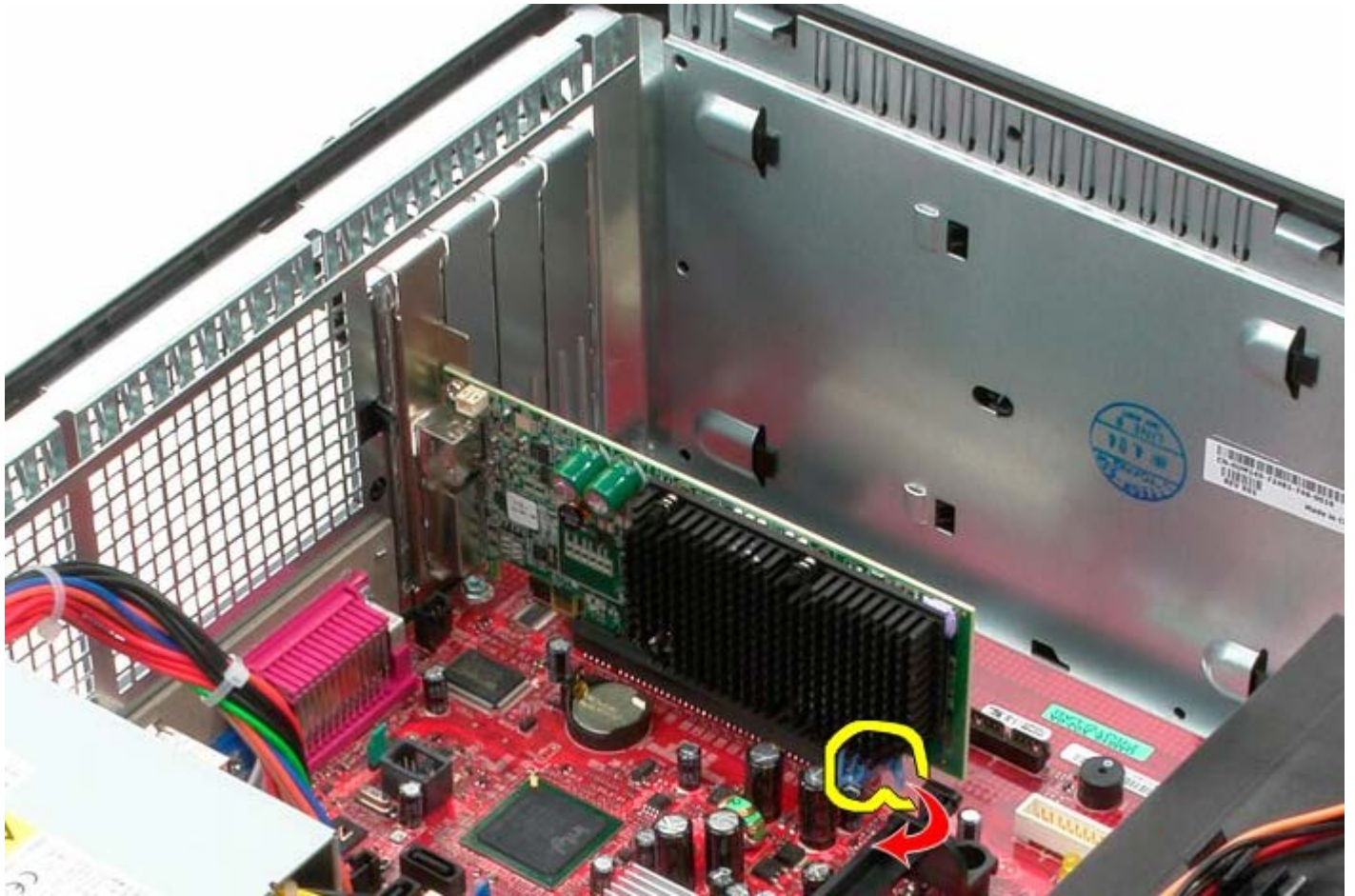
4. Angkat kartu ekspansi dan keluar dari slot ekspansi.
