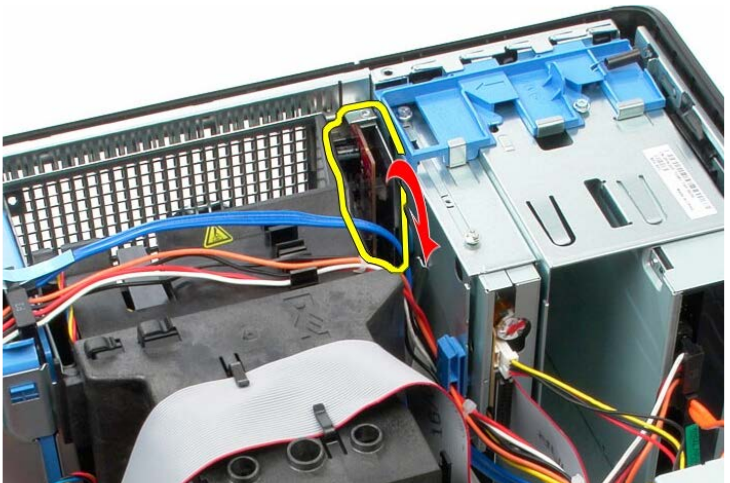
7. Angkat panel IO dari slotnya.
