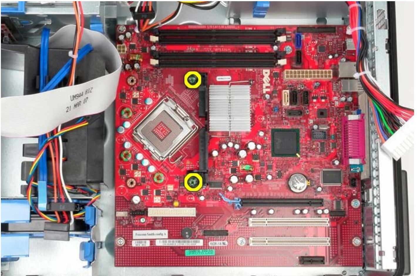
15. Lepaskan braket unit pendingin dari sistem.
