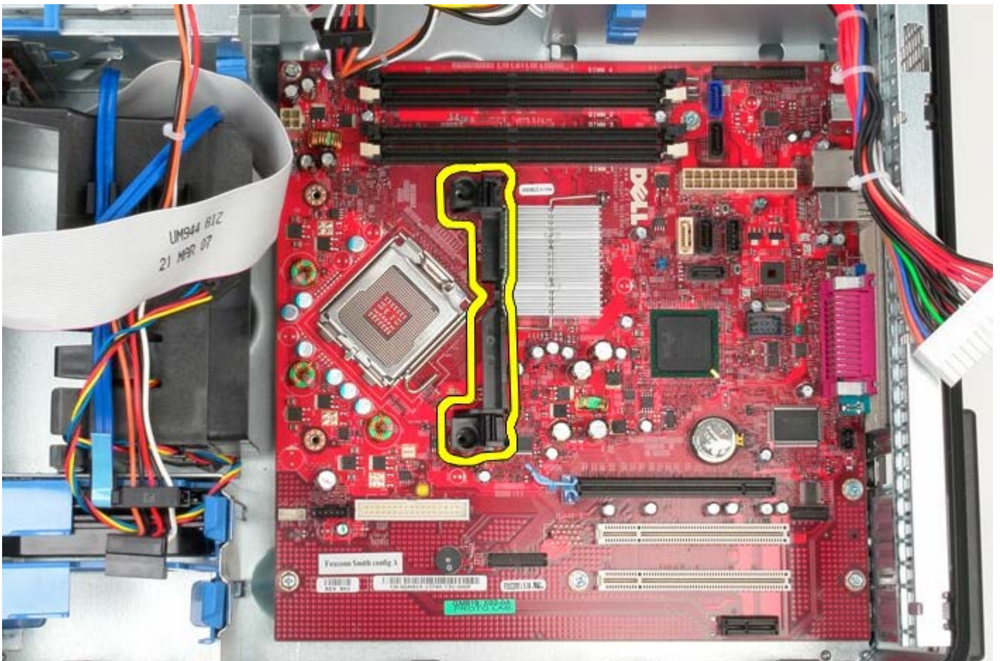
16. Lepaskan ketujuh sekrup yang menahan board sistem ke sasis.
