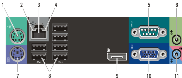
Figur 2. Visning af bagpanel
