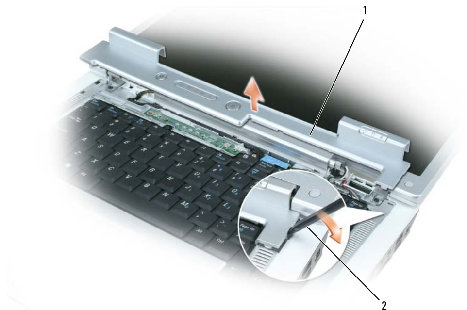
1 鉸接護蓋
