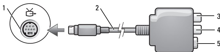
1 S-video 電視輸出連接器 2 合成式影像配接器 3 S/PDIF 數位音效連接器 4 合成式影像輸出連接器 5 S-video 連接器
