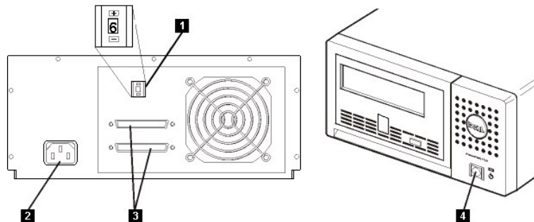
Figura 7. Panel trasero de la unidad de cintas externa
