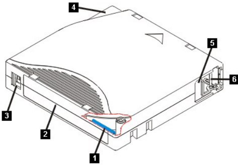
Figura 3. Cartucho de datos de LTO Ultrium de 400 GB
