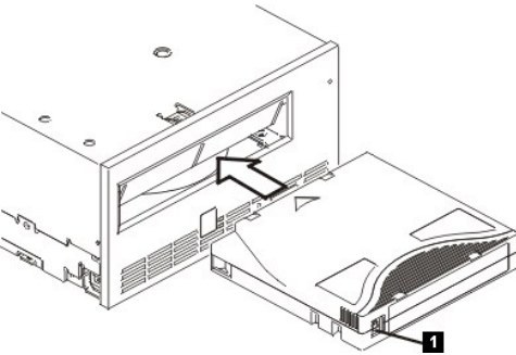
Figura 4. Cómo cargar
