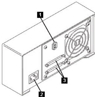
Figura 5. Panel trasero de la unidad de cintas externa
