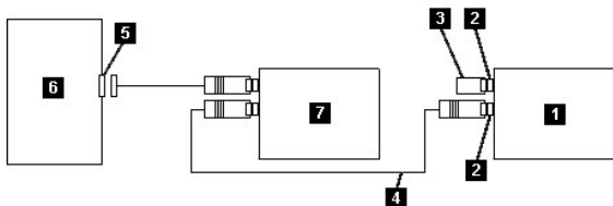
Figura 9. Conexión de varios dispositivos SCSI
