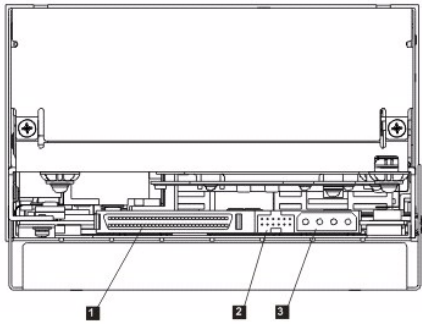
Figura 4. Panel trasero de la unidad de cintas interna
